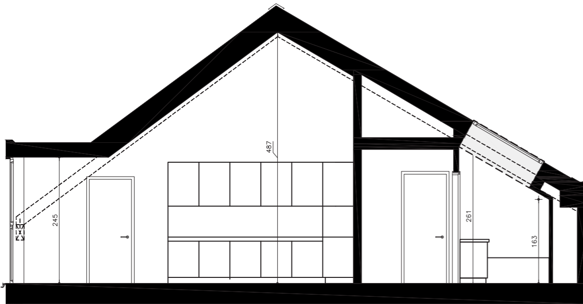
Doorsnede door leefruimte, keuken, nachthal en badkamer
