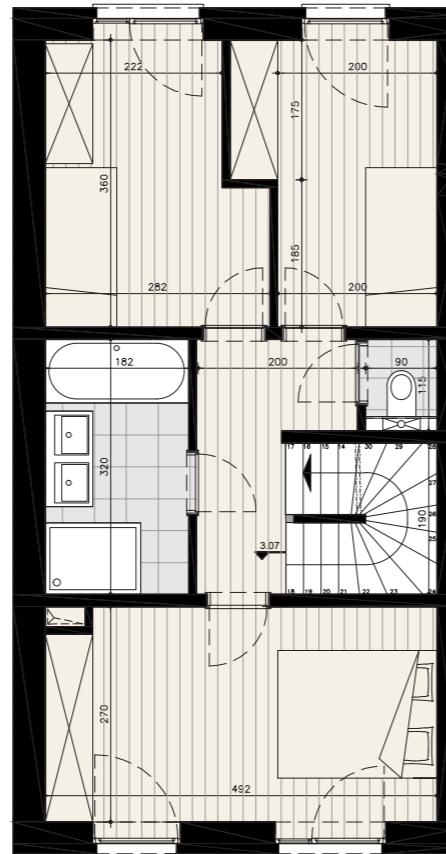
Verdieping +01
