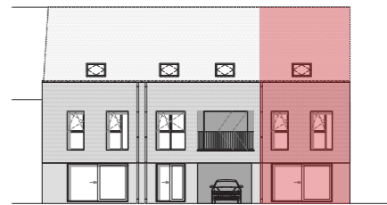
Achtergevel
